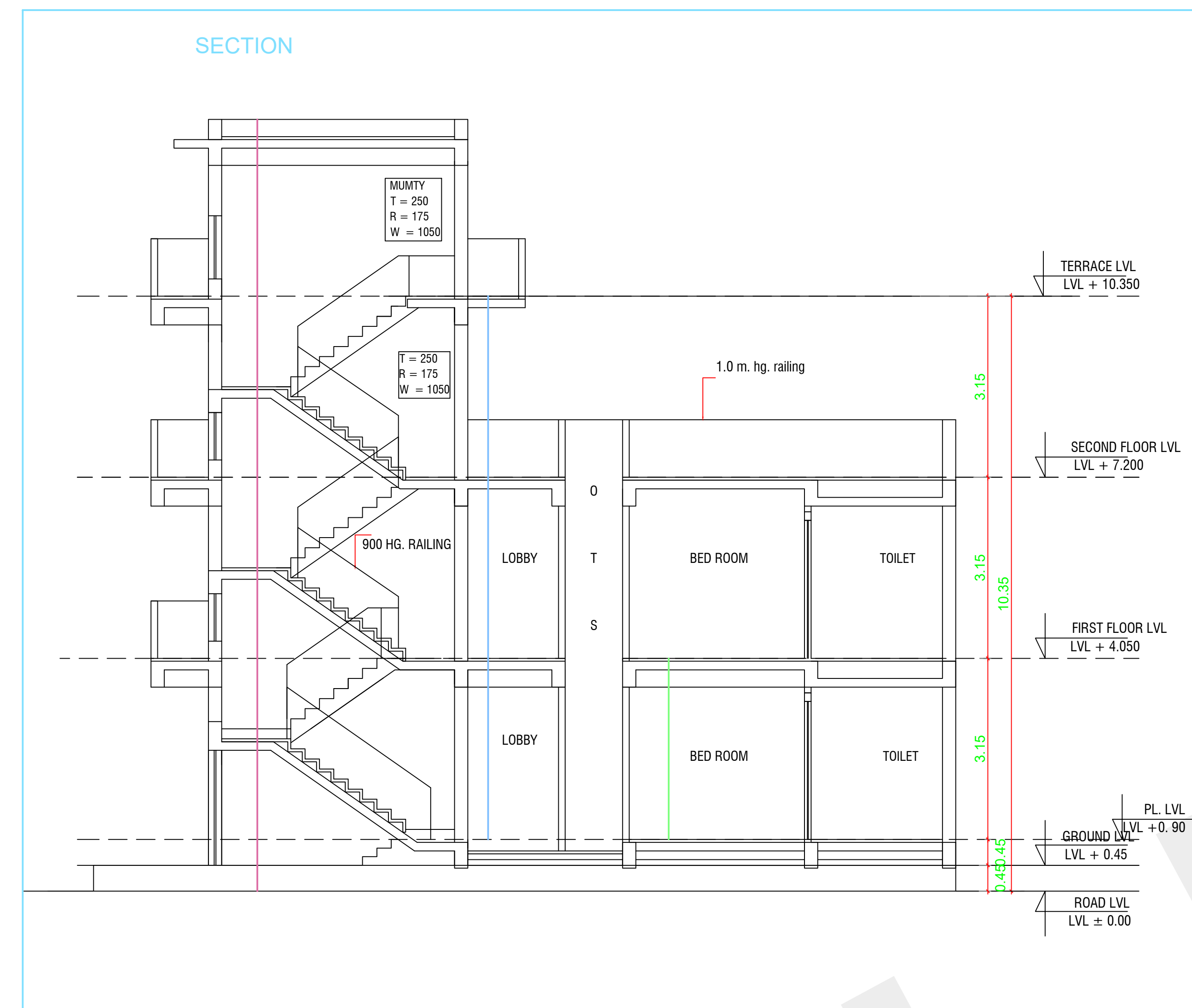
SECTION A-A
