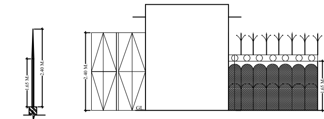
SECTION GATE(NTS.)
