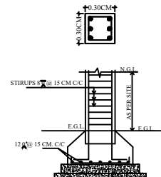
COLUMN DETAIL (SCALE : N.T.S.)
