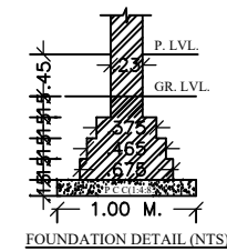
FOUNDATION DETAIL (N.T.S.)
